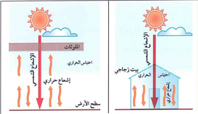
شكل (٣١) يوضح ظاهر حدوث الاحتباس الحراري في البيت الزجاجي وعلى سطح الأرض
